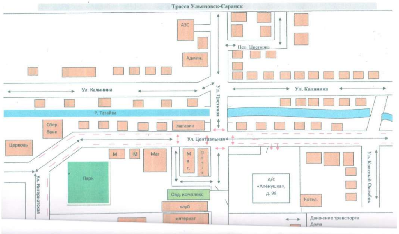
Схема организации дорожного движения в непосредственной близости от образовательного учреждения с размещением соответствующих технических средств, маршруты движения детей и расположения парковочных мест
